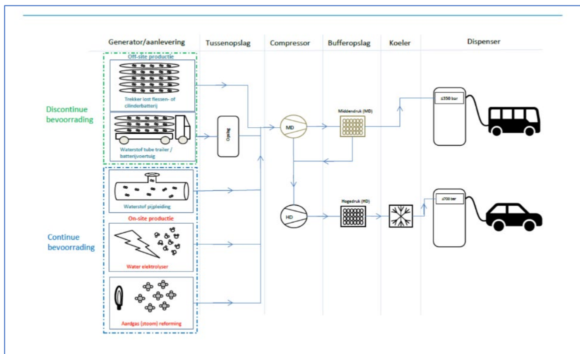
Figure 2. Hydrogen fueling station lay-out (ref. Kristof Custers, Philip Marynissen, Diane Huybrechts, Studie uitgevoerd door het Vlaams Kenniscentrum voor Beste Beschikbare Technieken (VITO), in opdracht van het Vlaams Gewest (2020).
